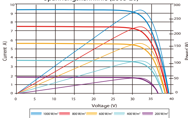
Strom-Spannungs- & Leistungs-Spannungskennlinie (280S-20)
