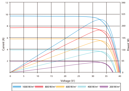
Strom-Spannungs- & Leistungs-Spannungskennlinie (295S-20)
